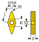
VNKG-M1
