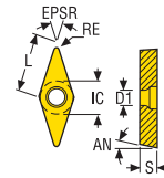
VBMT-MF2
