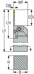
CFZR/L...JET/RBJET
